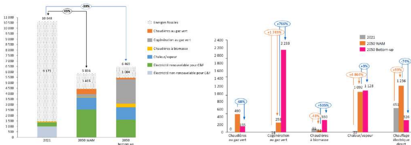
Figure 16 – Appvisionnement énergétique final par les combustibles fossiles et les énergies renouvelables pour 2021, 2050 WAM et 2050 Bottom-up (à gauche) et par technologie (à droite) [GWh]
