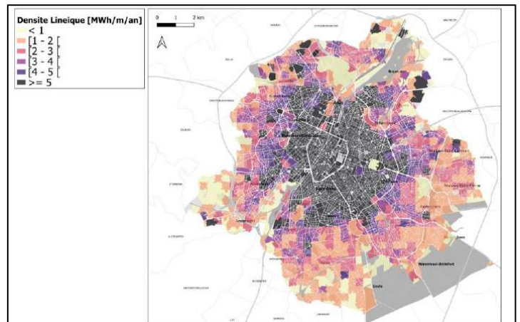
Figure 23 - Densité linéique des réseaux de chaleur
