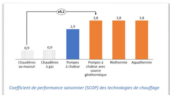
Figure 22 - Coefficient de performance saisonnier (SCOP) des technologies de chauffage
